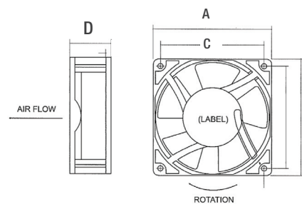
Dimensions - Frame Fan
