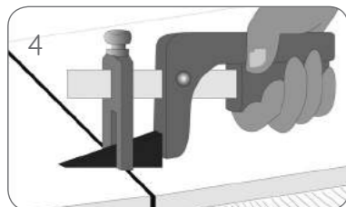
4 Apretar con el alicate especial. Grip with the ceramic pliers. Presser avec la pince spécial.
