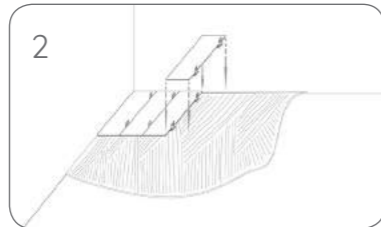
2 Colocación piezas cerámicas con los calzadores en las juntas. Installation of the pieces with the wedges at the edges. Pose des pièces avec les croisillons dans les joints.
