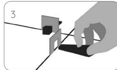
3 Colocación de las cuñas en los calzadores. Installation of the plastic wedges inside the cover wedges. Pose des cales en plastique dans les croisillons.
