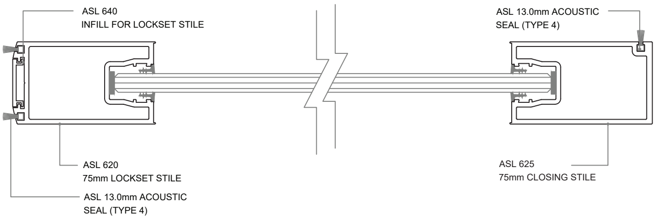
SLIDING DOOR
