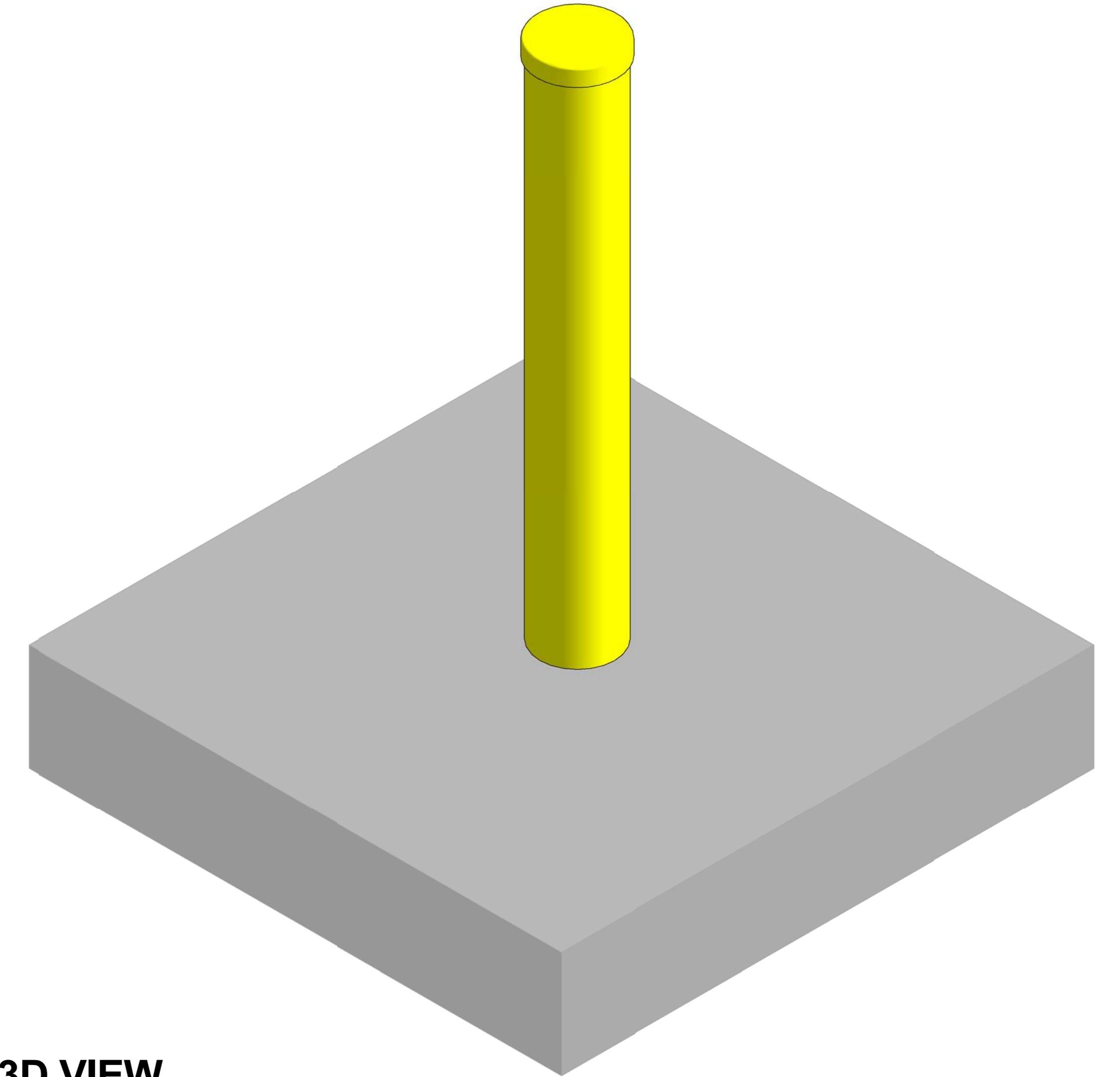
6 3D VIEW CAST-IN BOLLARD SCALE: N.T.S.
