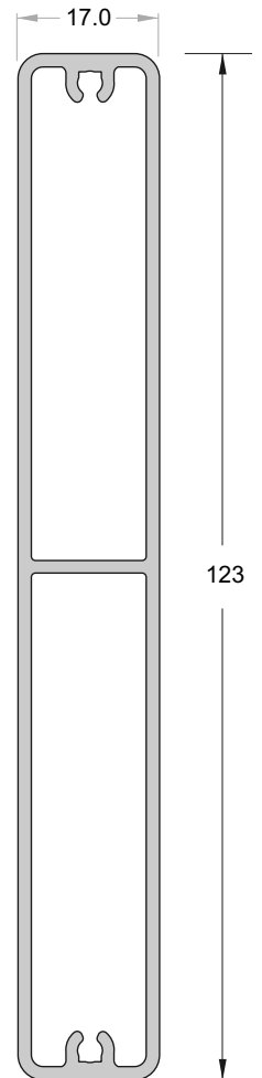
INFILL 123mm SLAT JGF/222/5.8
