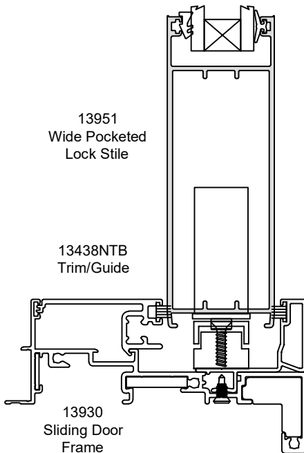
Optional Wide Stile
