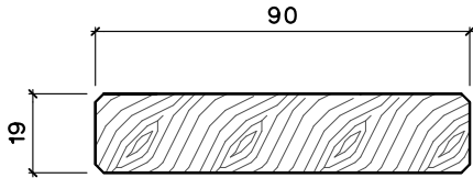
J4 Decking 90x19
