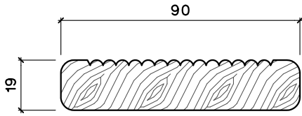
J3 Decking 90x19
