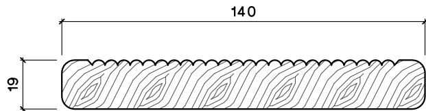
J5 Decking 140x19
