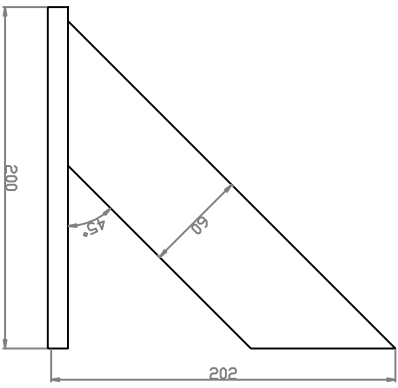
Elevation B Scale 1:1
