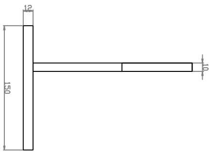
Elevation C Scale 1:1
