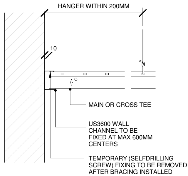
1 CEILING SEISMIC 1 : 5
